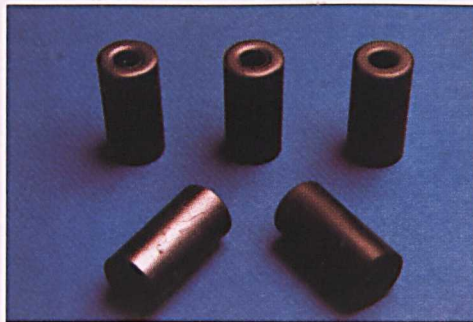
Selinder lompong sebagai penumpas gangguan elektromagnet
