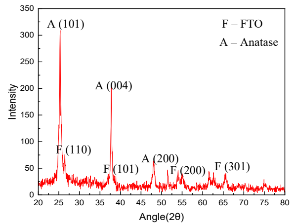
Fig. 2. XRD characterisation of TiO 2 on FTO.
