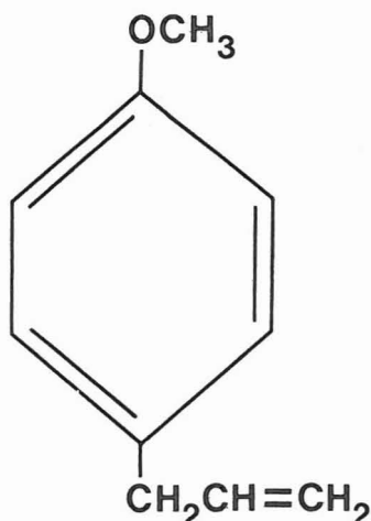
1-methoxy-4-(2-propenyl)benzene
